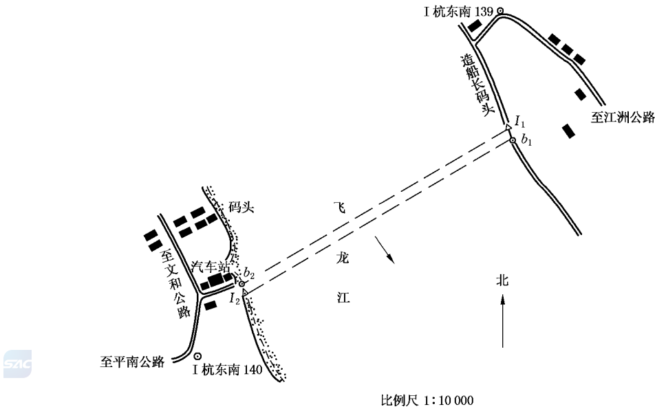
图 C.6 飞龙江跨河水准连测图
