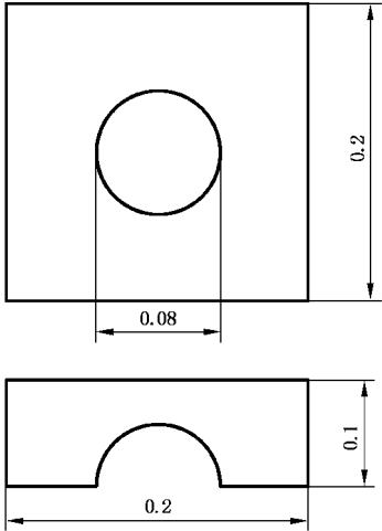
图 A.23 水准点标志盖
