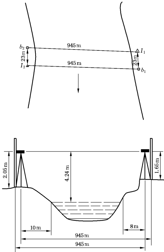
图 C.7 飞龙江跨河水准测量平、断面示意图
