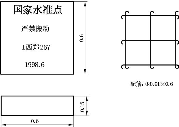
图 A.22 水准点保护盘
