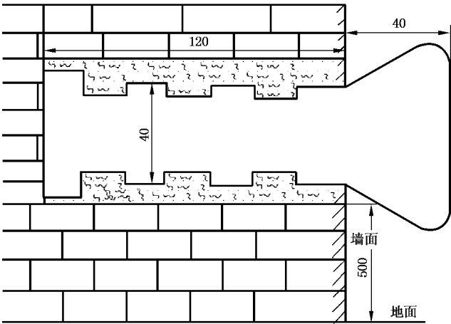
图 A.19 墙脚水准标志埋设图
