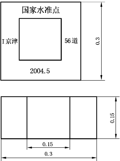
图 A.25 道路水准点保护框
