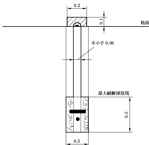
图 A.17 永冻地区钢管普通水准标石
