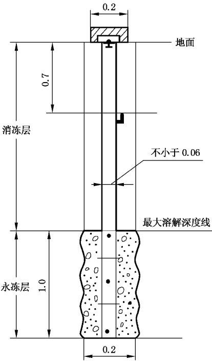
图 A.13 永冻地区钢管基本水准标石
