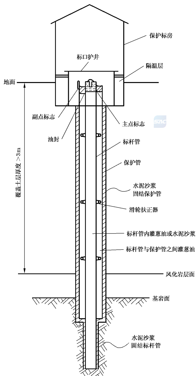
图 A.8 深层基岩水准标石示意图
