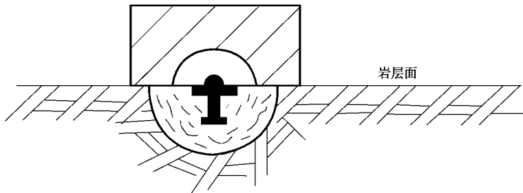
图 A.14 岩层普通水准标石
