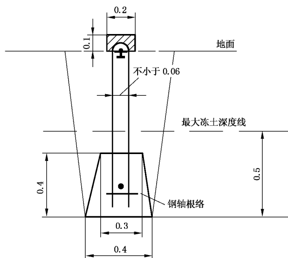
图 A.16 钢管普通水准标石
