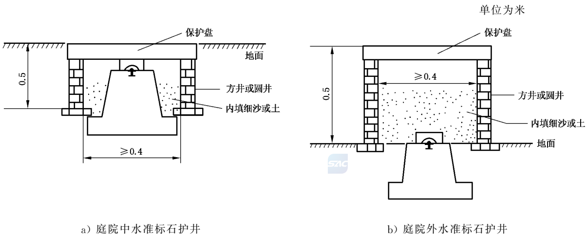
图 A.21 水准点保护井
