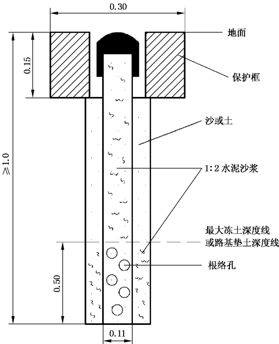
图 A.18 道路水准标石
